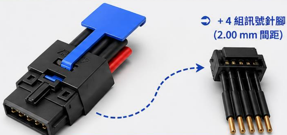
底部鎖扣式訊號模組 (Latch 結構)
